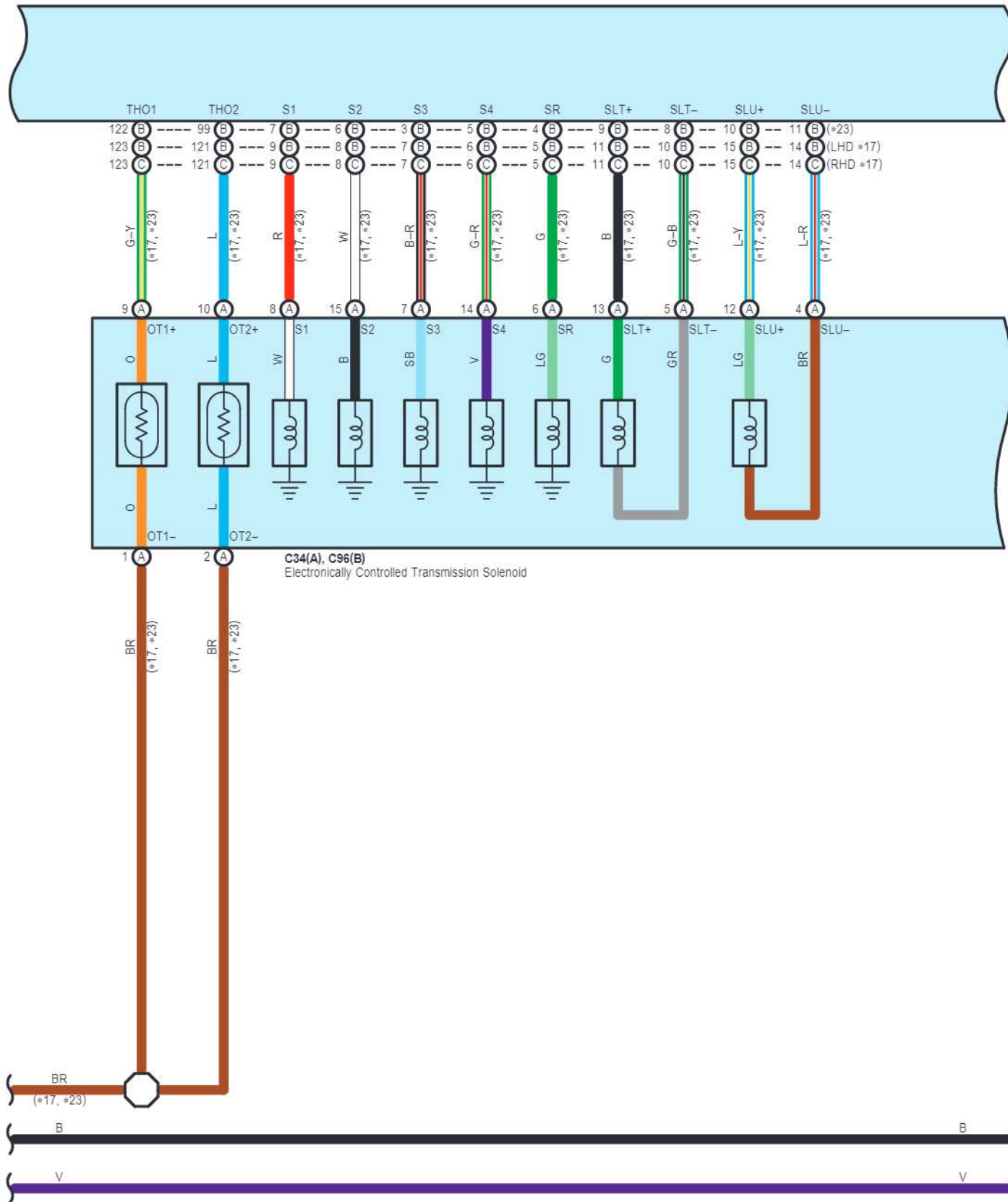
A38(A), A52(D), C45(B), C46(C) ECM
