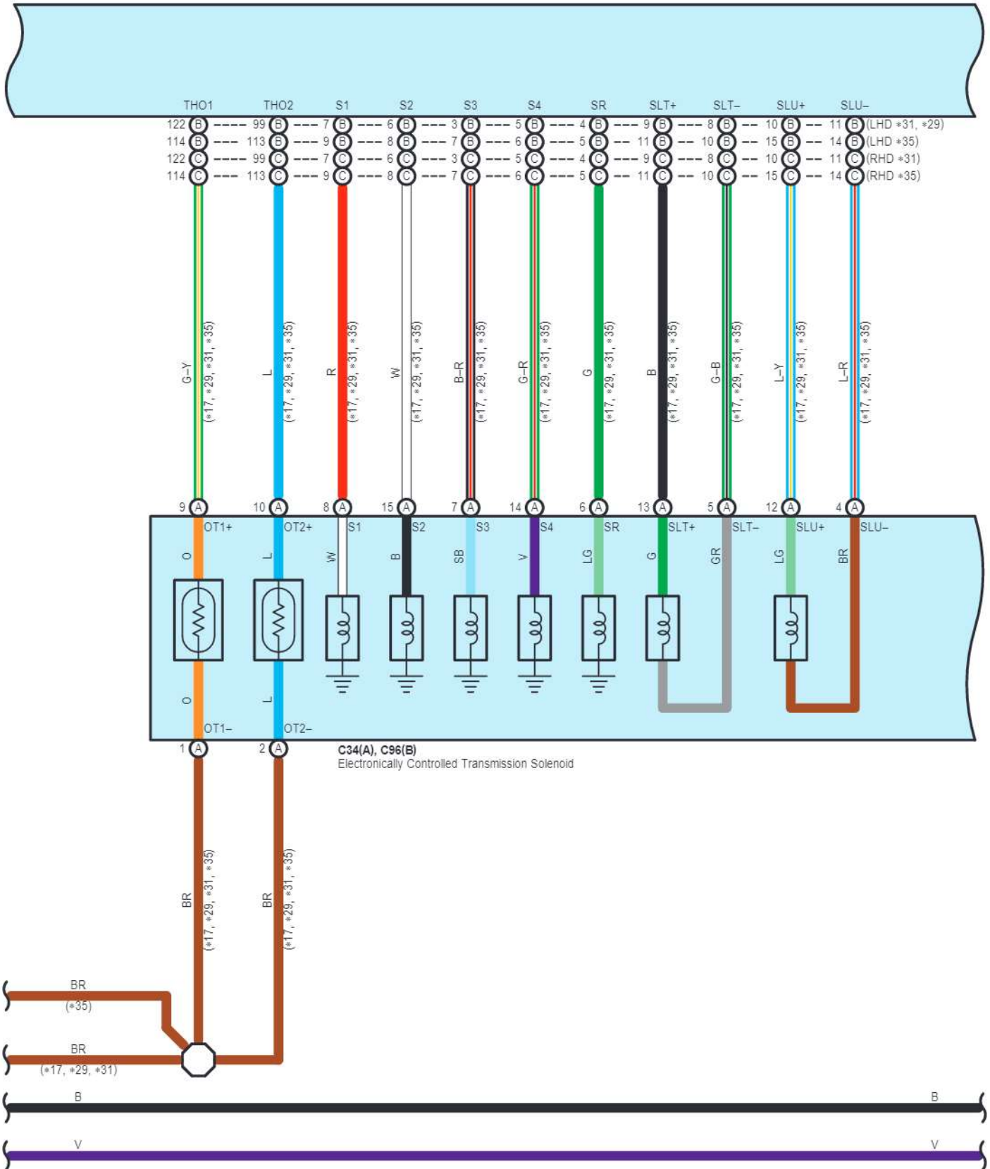
A38(A), A52(D), C45(B), C46(C) ECM
